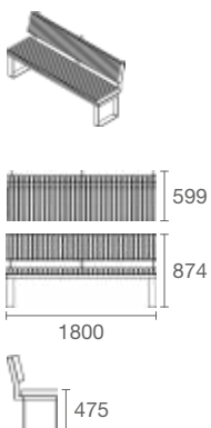
1 Module droit, avec dossier
